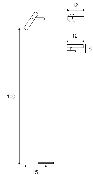
Gruppo lavabo con bocca da terra Floorstanding washbasin set
